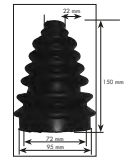
Fuelle Ø 95mm (4x4 furgonetas y grupo VAG)
